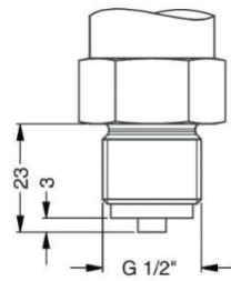
G1/2" EN 837-1/-3
